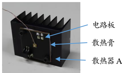
照片 2 评价光源的散热结构
