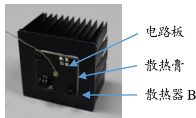
照片 3 评价光源的散热结构
